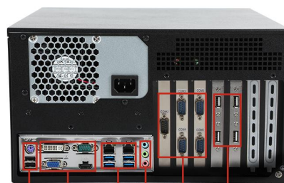
1*PS/2 1*DVI 2*USB2.0 1*VGA 1*HDMI 1*COM 3*音频接口 5*COM 4*USB2.0 2*千兆网口 4*USB3.0
