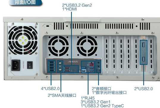
背面I/O图
