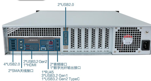
背面I/O图
