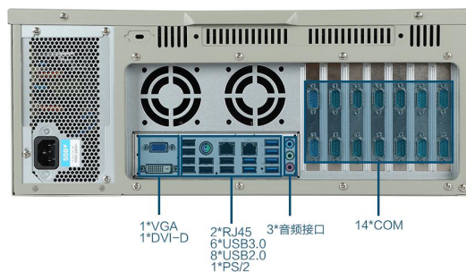
背面I/O图
