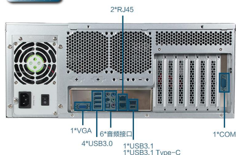
背面I/O图
