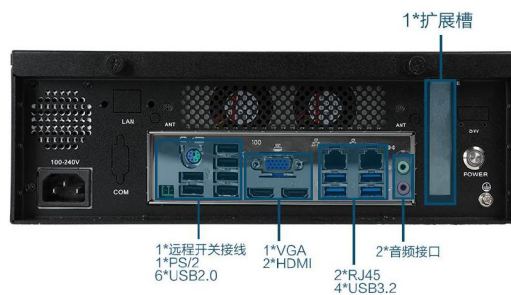
背面I/O图
