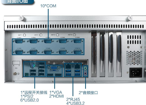
背面I/O图
