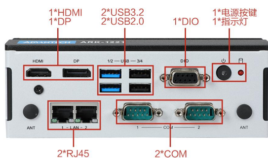
背面及安装尺寸图
