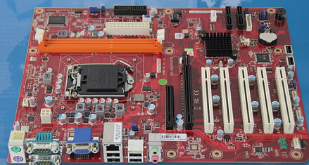
研华AIMB-701VG主板
