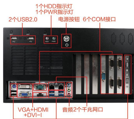
PS/2接口、4个USB2.0接口、4个USB3.0接口
